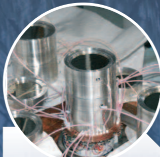
Physique nucléaire Nuclear physics
